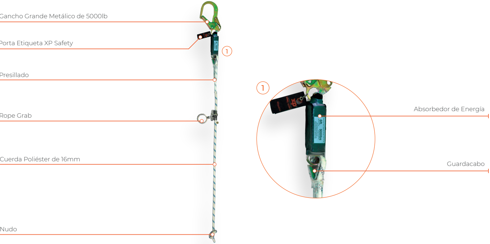
LÍNEA DE VIDA VERTICAL PORTÁTIL, CUERDA POLIÉSTER DE 16mm, CON GANCHO GRANDE, FRENO Y ABSORBEDOR DE ENERGÍA CERTIFICADO
